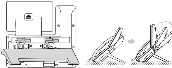
Tischinstallation
